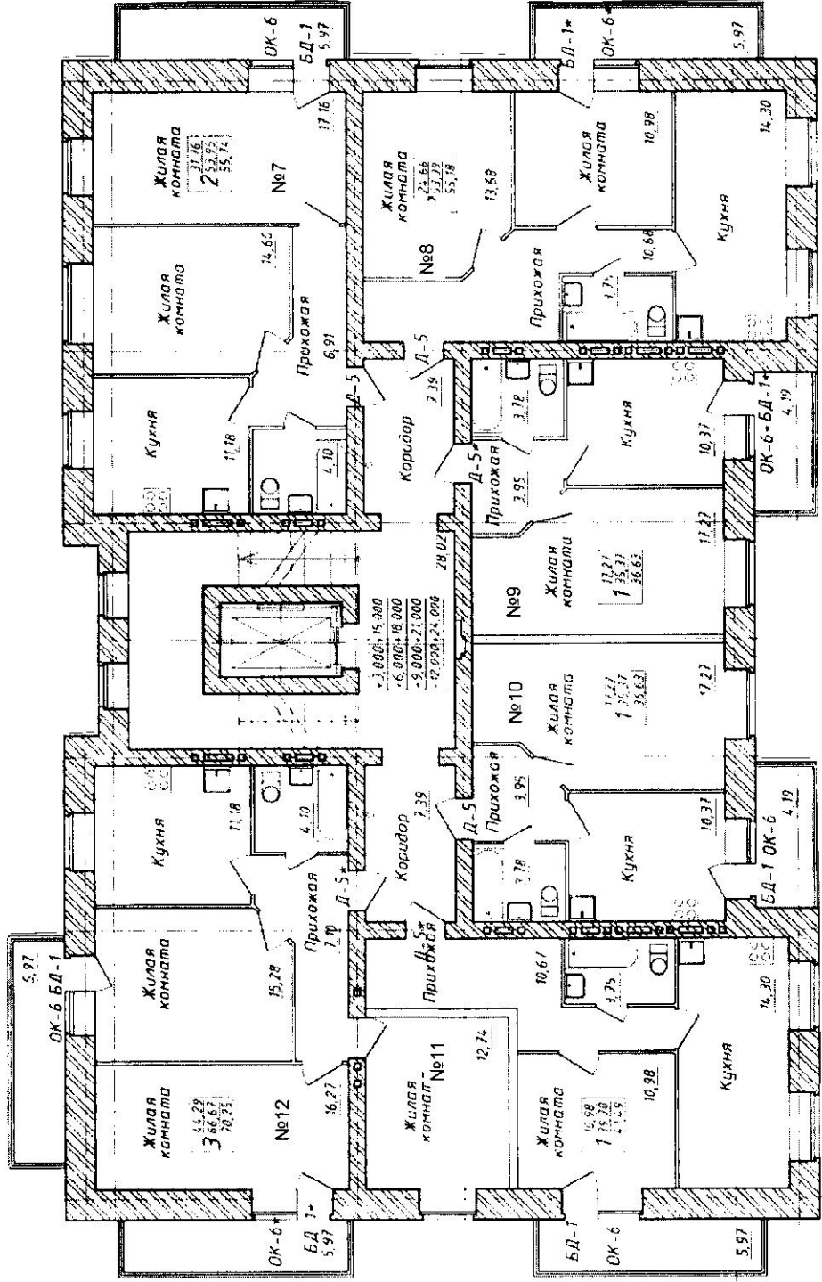
План 2-го этажа
